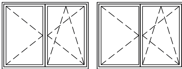
Drehfenster (DL) mit Stulp-Breit und Dreh-Kippfenster (DKR) Drehfenster (DL) mit Stulp-Schmal und Dreh-Kippfenster (DKR)
