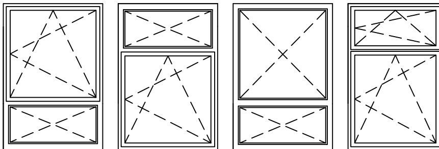
Dreh-Kippfenster (DKR) mit Unterlichte Fix Dreh-Kippfenster (DKR) mit Oberlichte Fix Fixfenster mit Unterlichte Fix Dreh-Kippfenster (DKR) mit Oberlichte Dreh-Kippfenster (DKR)
