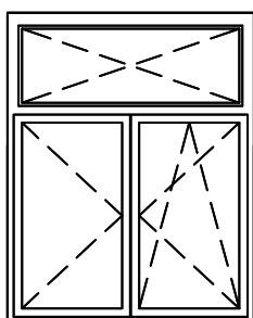
Drehfenster (DL) mit Stulp-Breit und Dreh-Kippfenster (DKR) mit Oberlichte Fix
