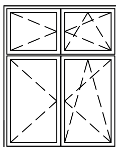
Drehfenster (DL) mit Stulp-Breit und Dreh-Kippfenster (DKR) mit Oberlichte Drehfenster (DL) mit Stulp-Breit und Dreh-Kippfenster (DKR)
