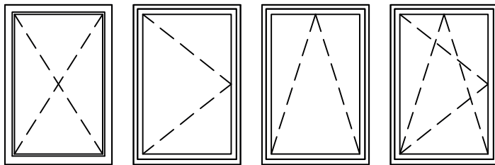
Fixfenster Drehfenster (DL) Kippfenster Dreh-Kippfenster (DKL)
