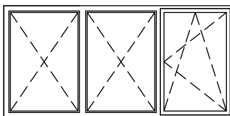
Fensterband (Fx-Fix-DKR)
