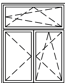
Drehfenster (DL) mit Stulp-Breit und Dreh-Kippfenster (DKR) mit Oberlichte Dreh-Kippfenster (DKR)
