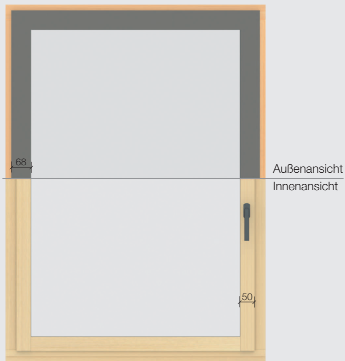
Holz/Alu Fenster HA-smal
