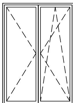
Balkontür mit Stulp (DL-DKR) in Standard und Nieder möglich 1)
